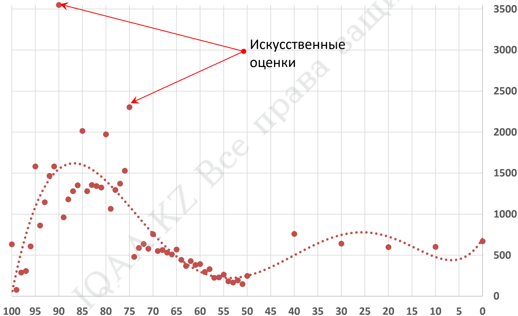
Распределение оценок осенней сессии университета 2017-2018 у.г. (выставлено 57867 оценок)
